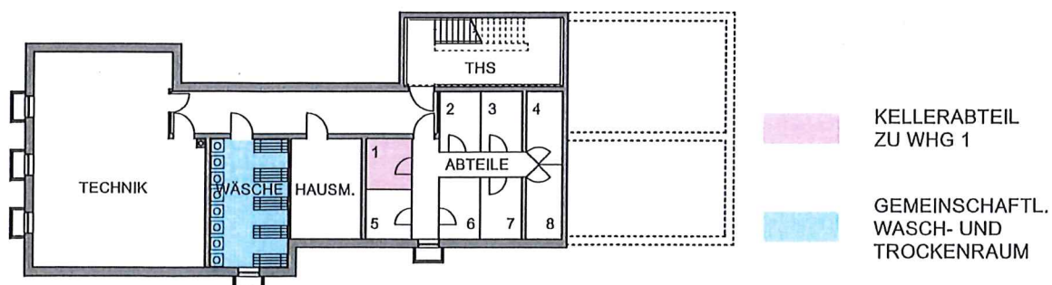
ÜBERSICHT KELLERGECHOSS
