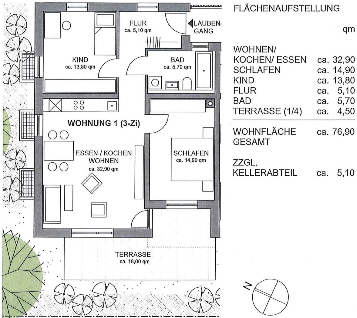
GRUNDRISS ERDGESCHOSS
